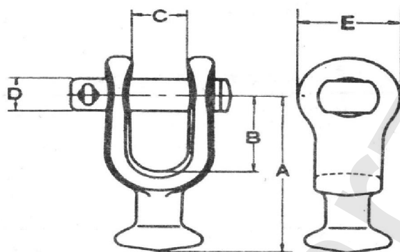
کلیس یا رکاب گوشتکوبی شکل (۵-۱): کلیس یا رکاب گوشتکوبی
