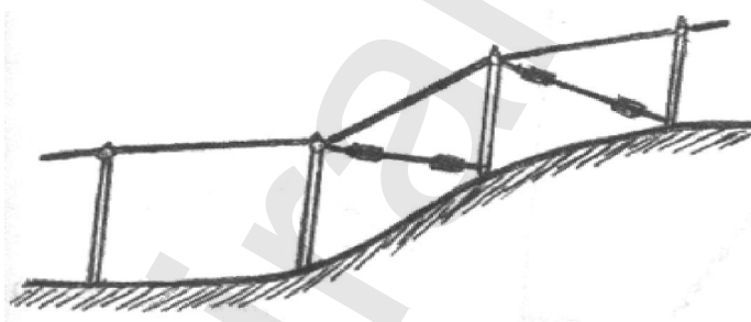
شکل ۲۸- مهار سر
