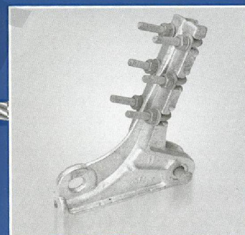
<< کلمپ انتهایی ۷۰ - ۳۵
