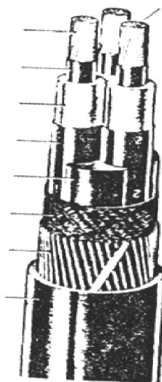
شکل ۳۰- الف - نمونه ای از کابل pex سه هسته 12-33\text{ kV}
