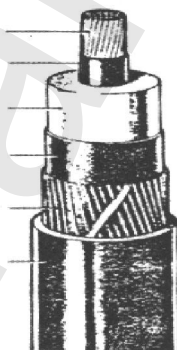
شکل ۳۰- ب- نمونه ای از کابل pex تک هسته 12-170\text{ kV}
