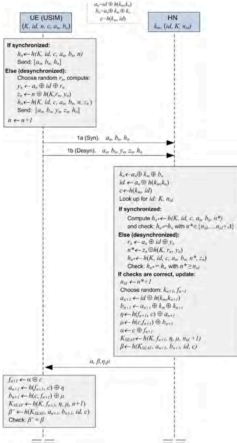
Fig. 3. The Braeken AKA protocol.
