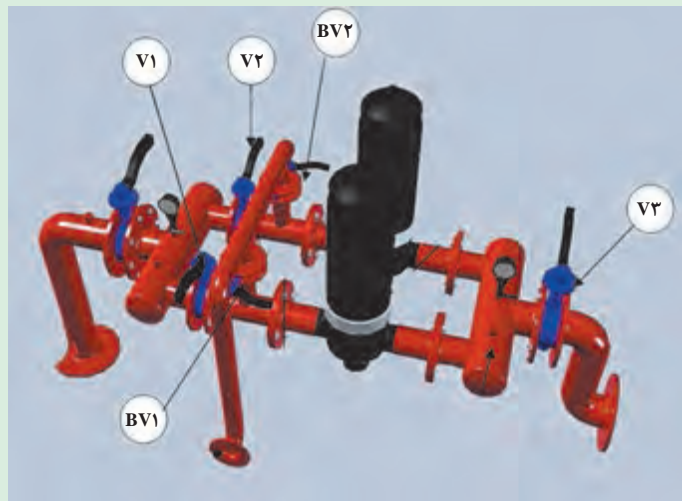
شکل ۶۱-۵. شیرهای روی صافی دوقلو دیسکی
