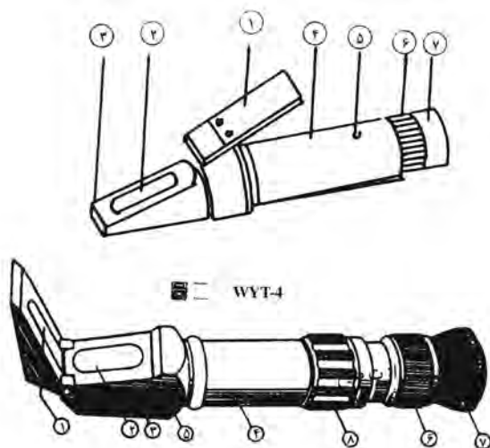
شکل ۳- رفاکتومترهای دستی
