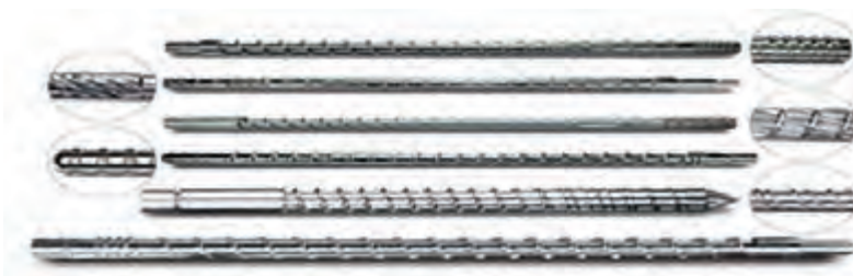
شکل ۱۱- انواع ماریپیچ برای ورز دادن خمیر در اکسترودر
