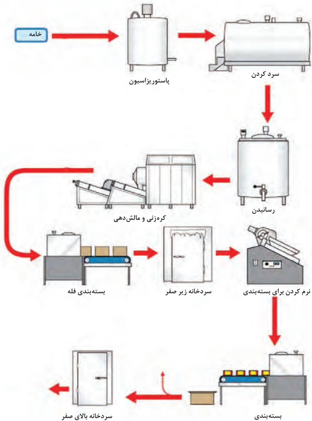
شکل ۵-۱۱- فرایند تولید کره
