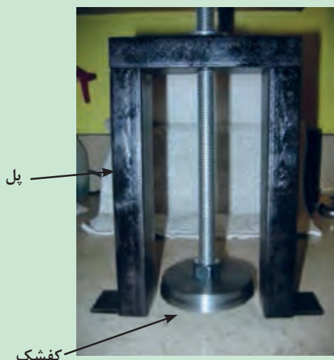
شکل ۵۵. خارج کردن بوش پیستون از بلوکه سیلندر با ابزار بوش کش
