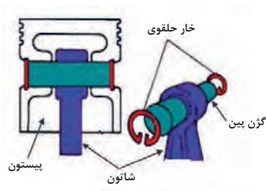
شکل ۱۵. اتصال شاتون به پیستون با گژن پین
