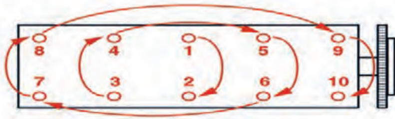
شکل ۳۹. بستن پیچ‌های سرسیلندر به روش حلزونی
