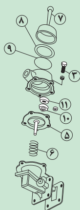
شکل ۳۷. شکل شماتیک و نمای برش خورده پمپ مقدماتی تراکتور MF285
