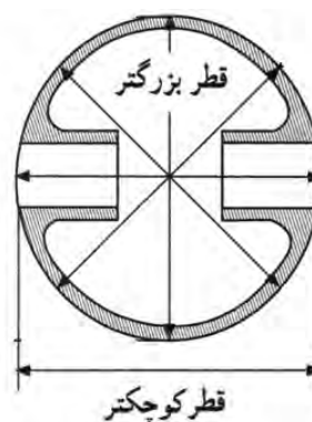
شکل ۷. اندازه قطرهای پیستون
