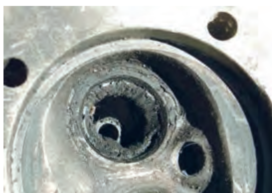
شکل ۶۷. کربن گرفتگی سرسیلندر و سوپاپ‌ها
