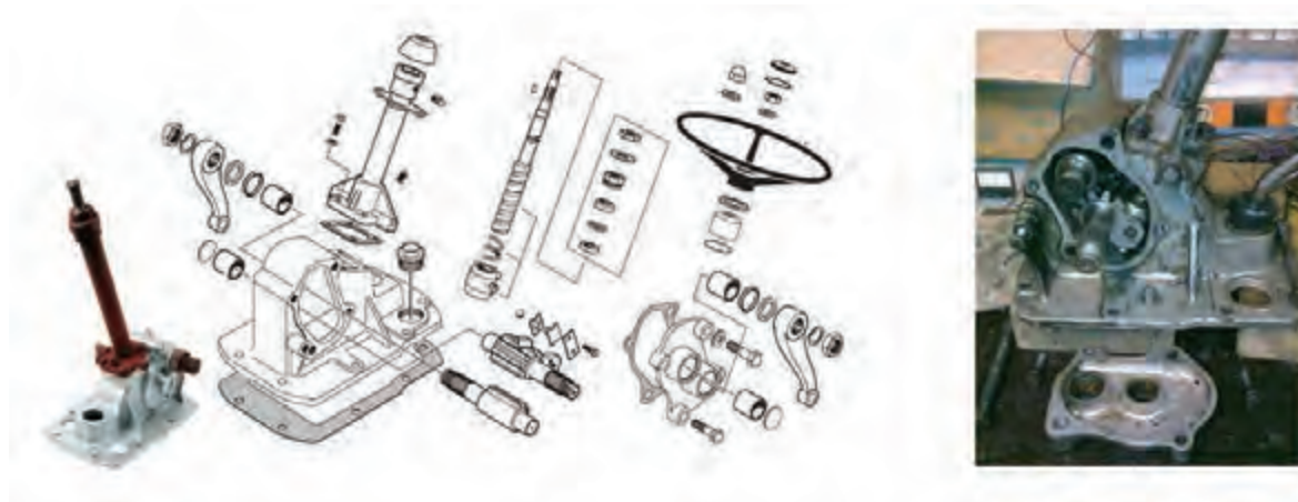
شکل ۱۳. جعبه فرمان تراکتور U650M
