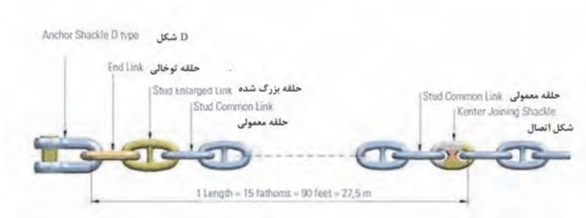
شکل ۳-۵- نحوه قرار گرفتن شکل‌ها و حلقه‌ها در یک طول زنجیر لنگر
