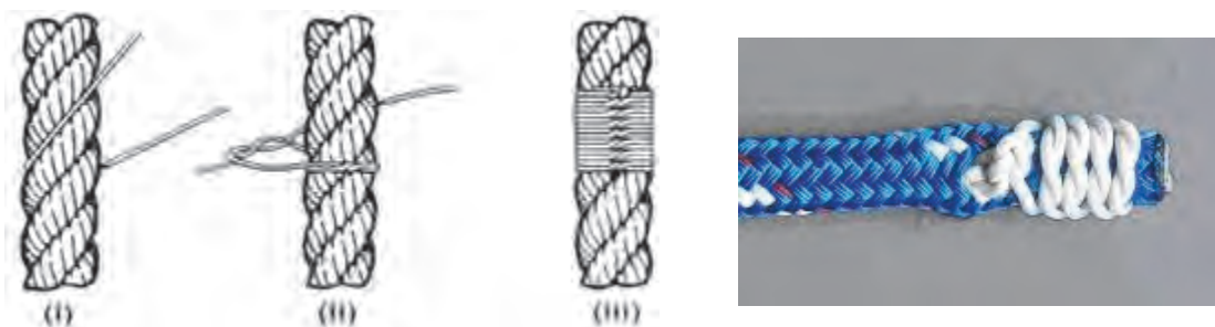
شکل ۲-۲۳- نخ پیچی غربی
