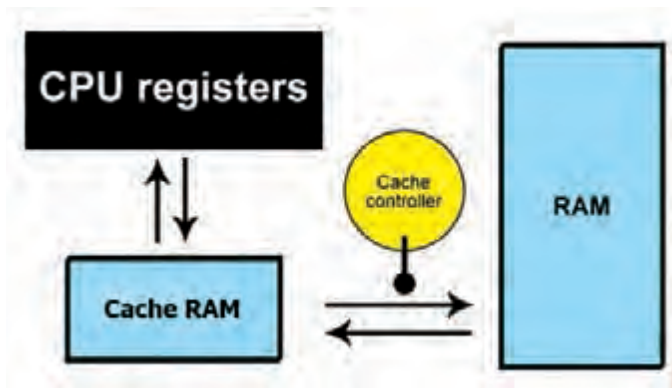
شکل ۱۸- ارتباط حافظه نهان و ثبات با RAM
