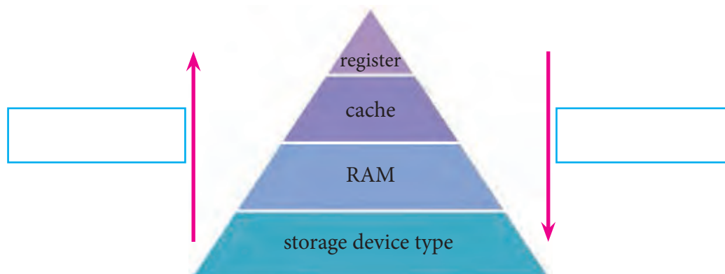
شکل ۲۰- هرم حافظه
