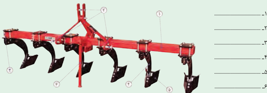
شکل ۱۳- ساختمان شیارکش
