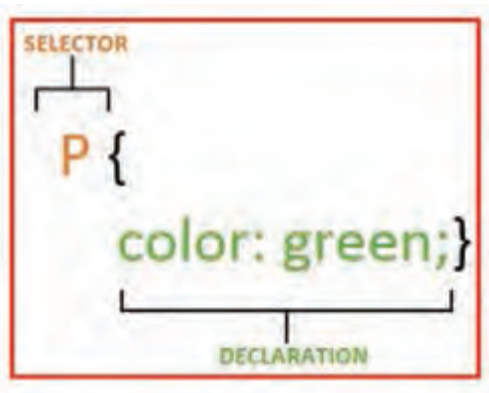
شکل ۱۳- بخش‌های مختلف یک قانون در CSS
