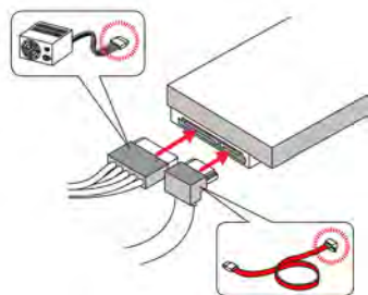
شکل ۴۹- اتصال کابل داده و تغذیه دیسک سخت
