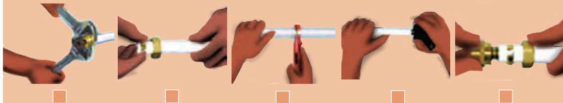
شکل ۴۴- مراحل اتصال لوله پکس
