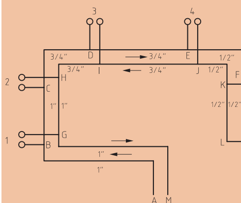
شکل ۱۴- نقشه کار لوله‌کشی برگشت مستقیم
