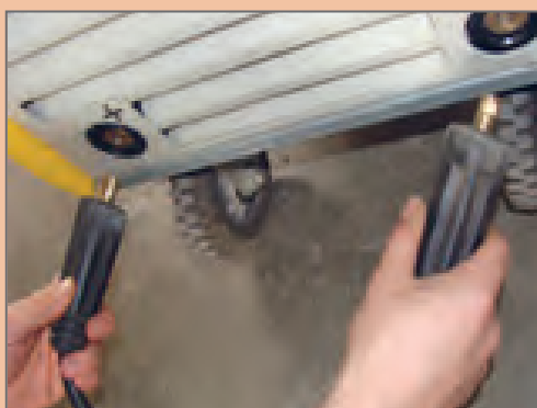
شکل ۴۰- اتصال انبرها
