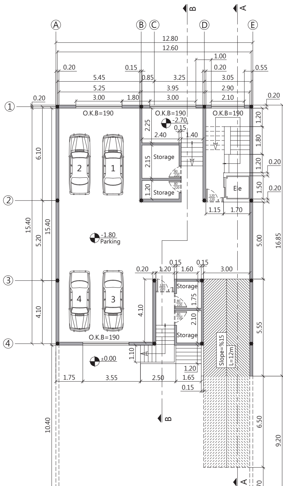
شکل ۷- پلان طبقه همکف
