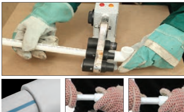
شکل ۵۶- مراحل اتصال PPR
