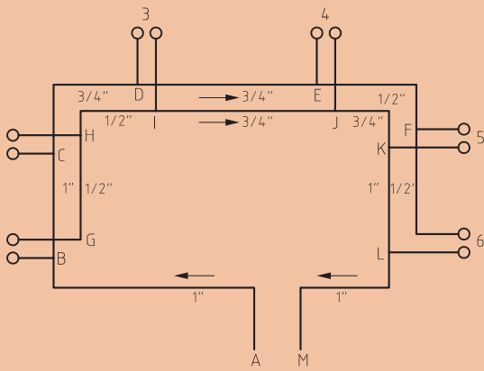
شکل ۱۵- نقشه کار لوله‌کشی برگشت معکوس
