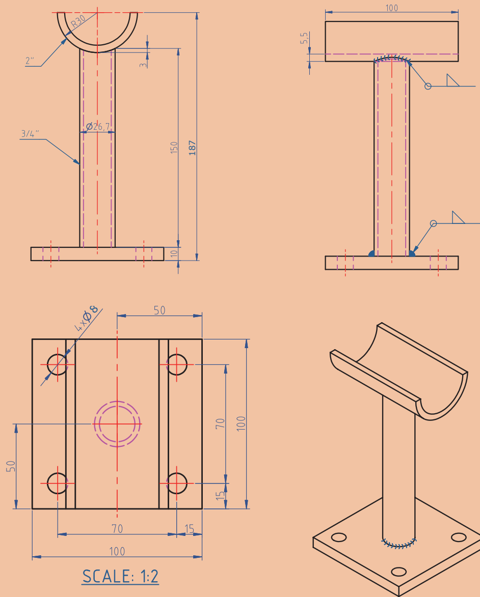
شکل ۵۴- نقشه کار ساخت خرک
