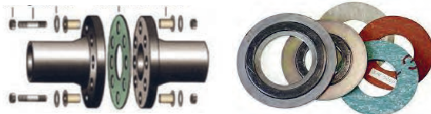
شکل ۳۴- انواع واشر آب‌بندی
