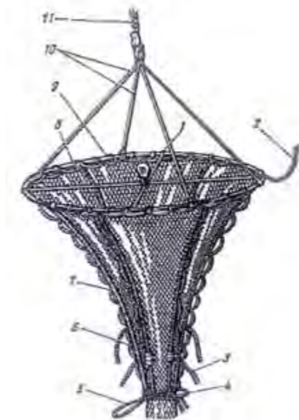
شکل ۴۲- اجزا و متعلقات یک تور قیفی (۱- لامپ، ۲- کابل برق، ۳- طناب کوتاه کمربندی، ۴- حلقه‌های فلزی، ۵- طناب بستن ته تور، ۶- وزنه یا زنجیر، ۷- طناب طولی تقویت کننده بدنه تور، ۸- طناب‌های صلیبی، ۹- حلقه فلزی دهانه تور (قاب فلزی)، ۱۰- طناب‌های نگهدارنده تور، ۱۱- کابل وینچ
