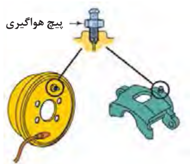
شکل ۹-۶- جای قرارگیری پیچ هواگیری روی سیلندر ترمز چرخ
