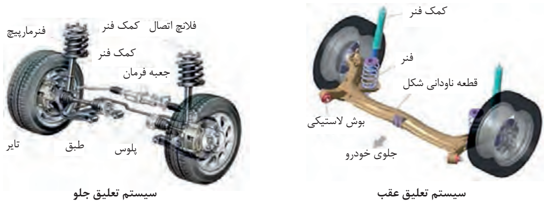
شکل ۱-۲۹- نمونه‌هایی از سیستم تعلیق و اجزای آن
