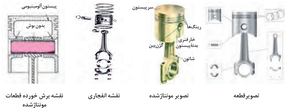
شکل ۵-۸- انواع تصوير و نقشه
