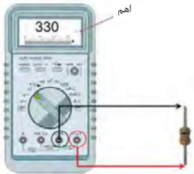
شکل ۱۲-۷- اندازه‌گیری مقاومت
