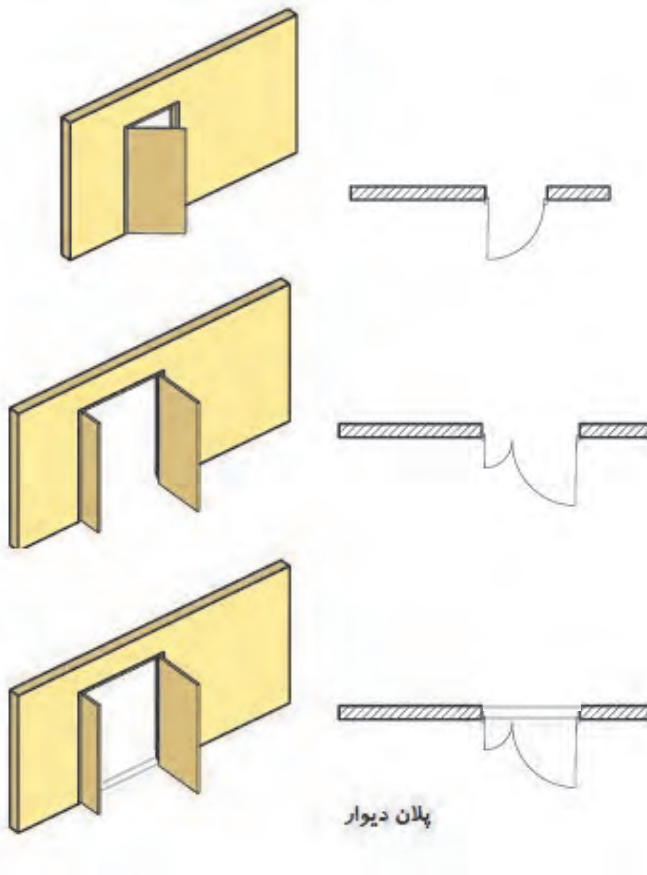
شکل ۲۲ ترسیم درها در پلان
