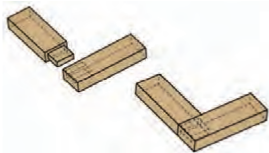
شکل ۱۷- تصویر سه بعدی از اتصال کام و زبانه گوشه‌ای (مخفی)
