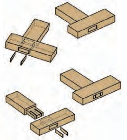
شکل ۱۹- اتصال کام و زبانه با دو شیار روی زبانه و دو گوۀ چوبی که درون شیارها قرار می‌گیرند.
