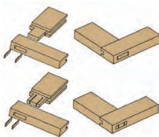
شکل ۱۸- اتصال کام و زبانه با دو گوۀ چوبی در دو طرف زبانه
