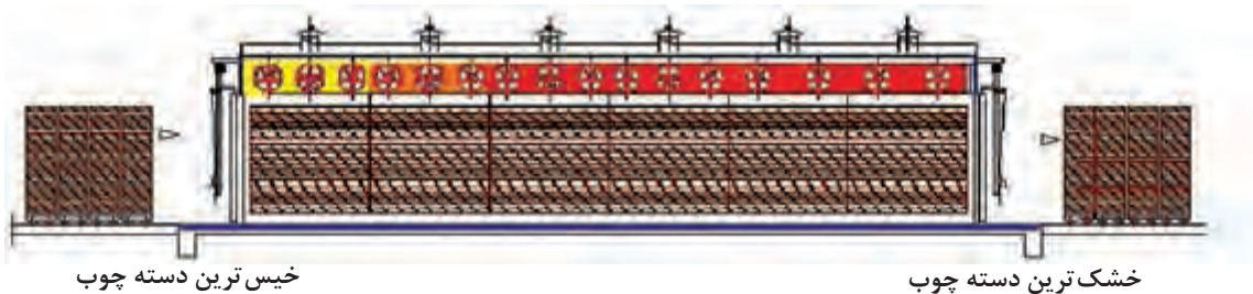
شکل ۲۶- کوره پیوسته چوب خشک‌کنی مجهز به سیستم جریان اجباری هوا
