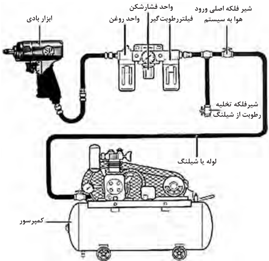
شکل ۴۵- نمونه‌ای از یک سیستم ساده هوای فشرده و ابزارهای بادی
