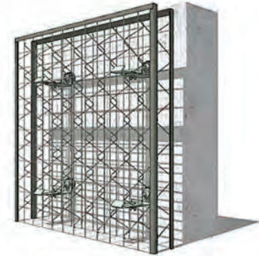
پانل فلزی در سیستم شبکه‌ای داربستی
