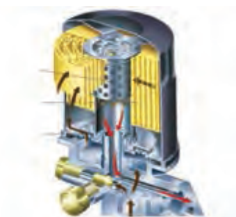
سوپاپ کنار گذر روغن
