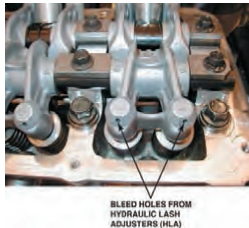
اسبک دوپل با تنظیم کننده هیدرولیکی
