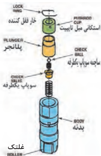
تایپیت غلتنکی با تنظیم کننده هیدرولیکی در موتور OHV
