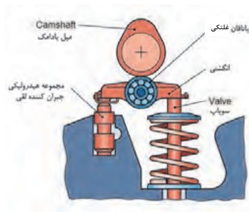
تایپیت با تنظیم کننده هیدرولیکی در موتور OHC-OHV
