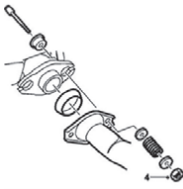
انفجاری گلوبی آگزوز
