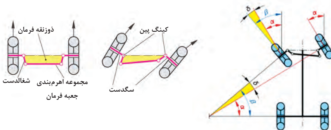
شکل ۱۲- هندسه فرمان
