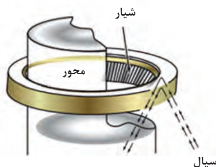
شکل ۸- کاسه نمد با لبه شیاردار
