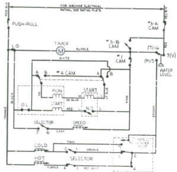
نقشه لباسشویی جنرال مدل: (090) 96 D 560
