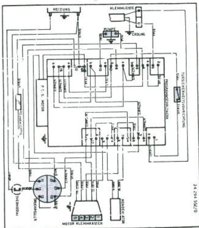
نقشه لباسشویی آ.ا.گ لاوالوکس
