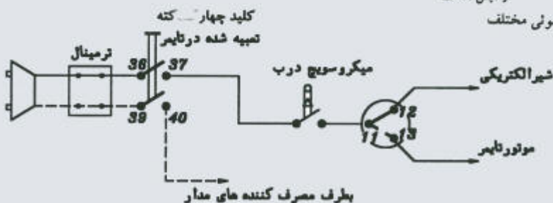
تسمتی از مدار سیم بندی ماشین آزمایش مدل ۲۰۰۱
