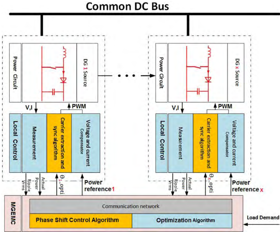
Fig. 1. DCMG scheme.
