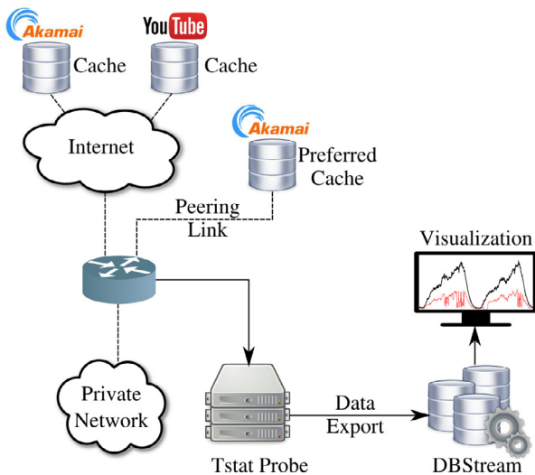
Fig. 5. Tstat plus DBStream.
