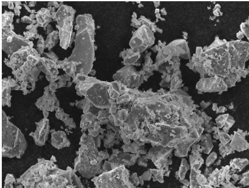
cal_0011 2015/04/30 NMU x1.5k 50 μm Università di Udine
