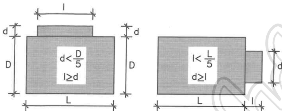
شکل ۷-۱ ابعاد پیش‌آمدگی در پلان ساختمان
