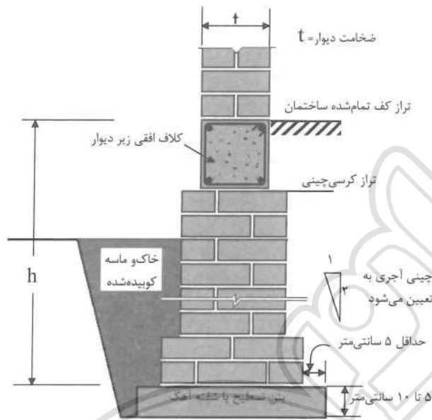
شکل ۶-۷ شالوده متشکل از مجموع کلاف افقی زیر دیوار و کرسی چینی آجرچینی
