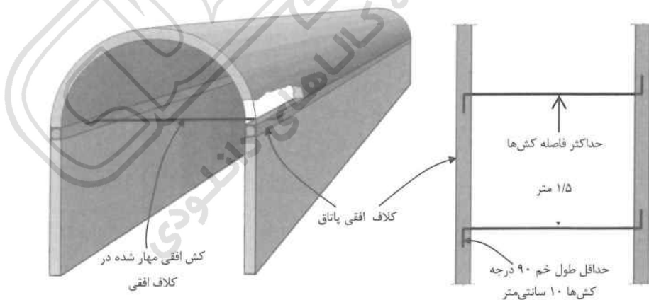
شکل ۷-۳۱ تعبیه مهاربندهای افقی در پاتاق‌های قوسی استوانه‌ای
