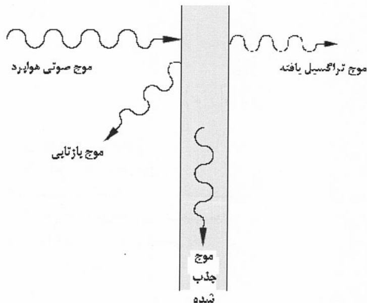
شکل ۱۸-۱-۳: تراگسیل صدای هوابرد از طریق یک جداکننده
