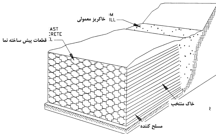
الف) مسلح کننده تسمه فلزی با نمای پانلی
