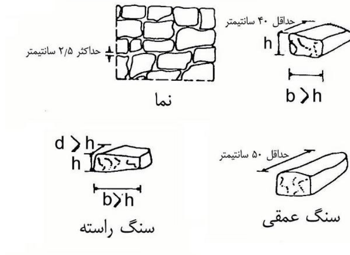
شکل ۵-۱ بنایی با سنگ قواره Moellon Brut (UR) Uncoursed Rubble Masonry
