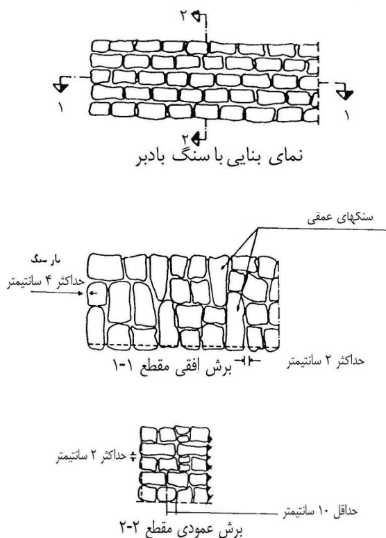
شکل ۳-۵ بنایی با سنگ بادبر Coursed Rubble Masonry
