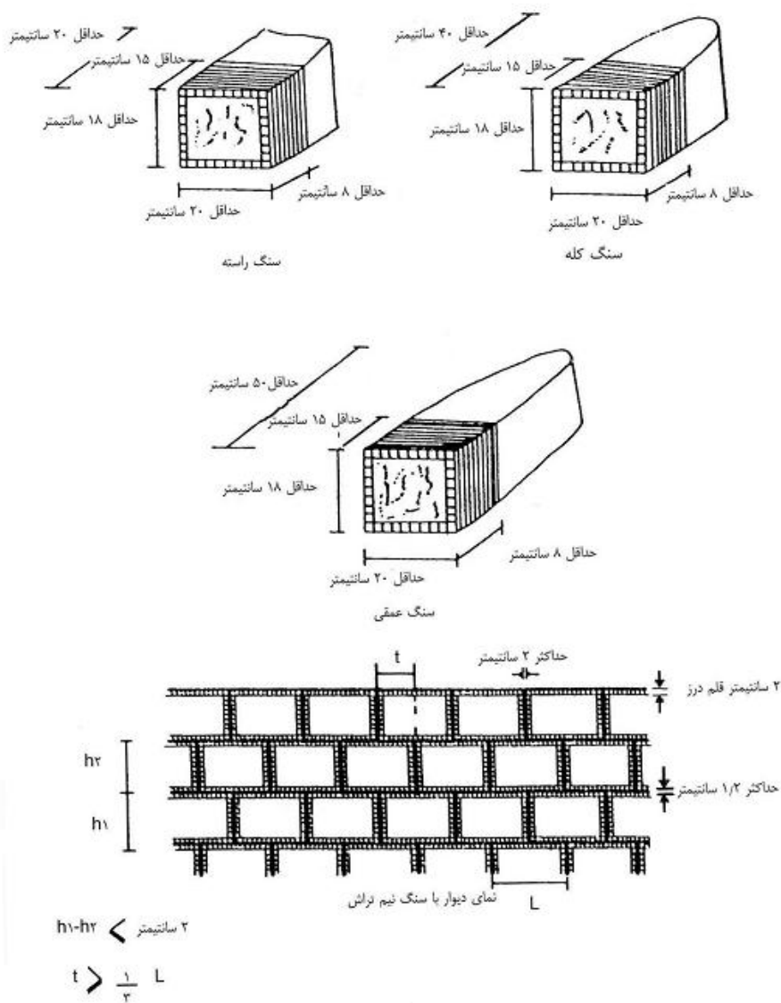
شکل ۵-۶ بنایی با سنگ نیم سرتراش Moellon Pique
