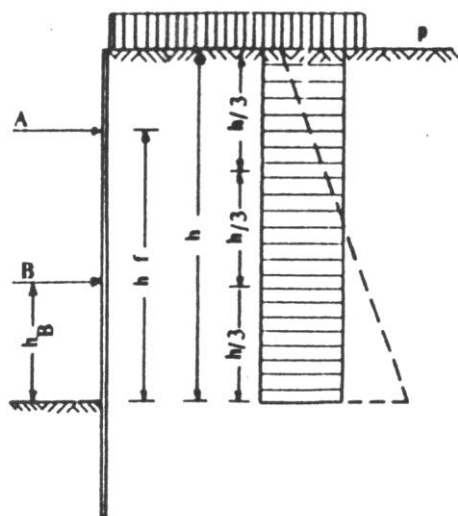
شکل ۶-۸ سپر دارای دو تکیه‌گاه یا دو مهار
