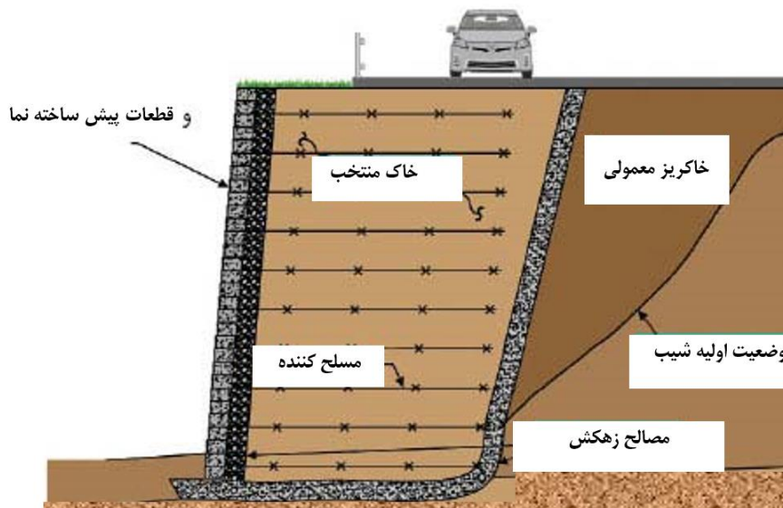
ب) مسلح کننده ژئوگریدی با نمای بلوک مدولار بتنی
