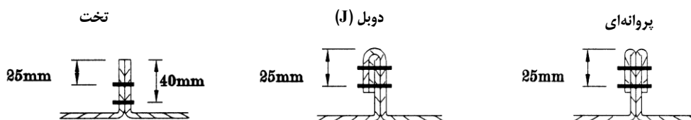
شکل ۲۲- ۲ سه نوع متداول درز
