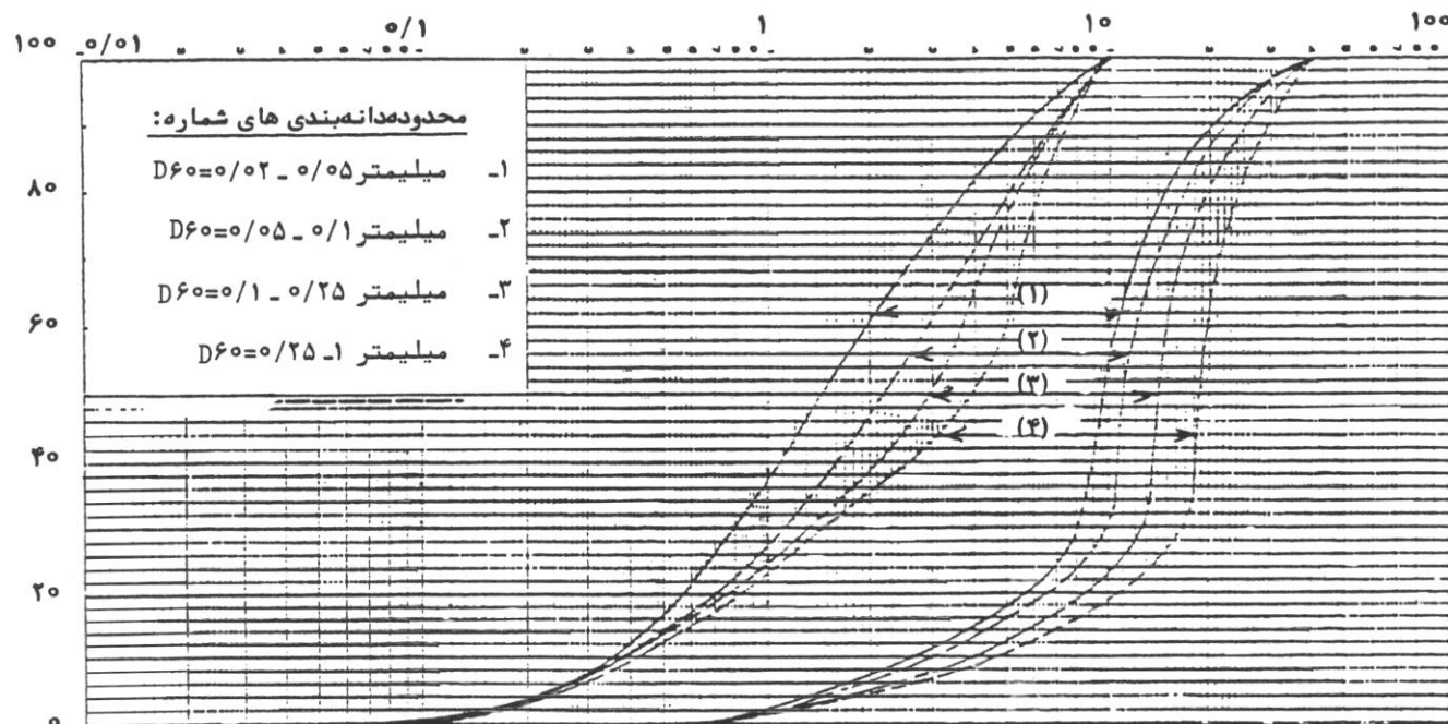
شکل ۱۱-۲ محدوده دانه بندی مصالح فیلتر برای انواع خاک پایه با D_{60} از ۰/۰۲ تا ۱ میلی متر
