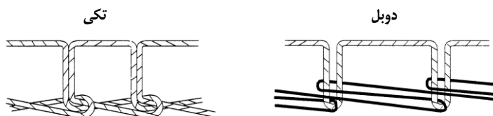
شکل ۲۲- ۱ دو نوع کوک‌زنی (تکی و دوبل)
