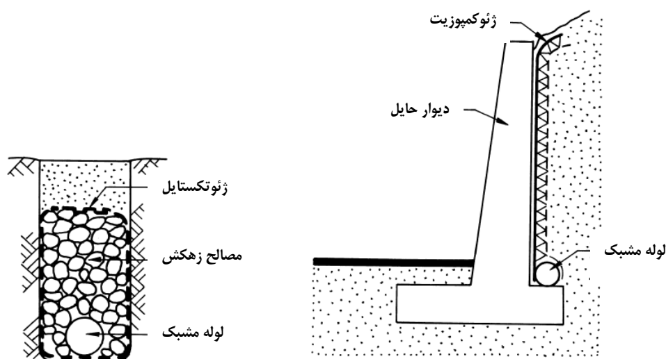
عملکرد فیلتراسیون ژئوتکستایل در کانال زهکشی
