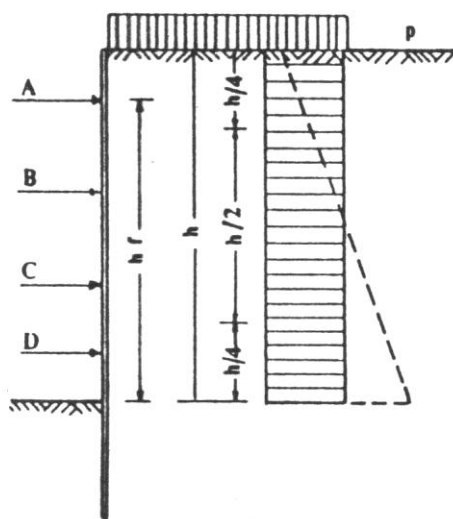
شکل ۶-۹ سپر دارای سه یا تعداد بیشتری تکیه‌گاه یا مهار باشد
