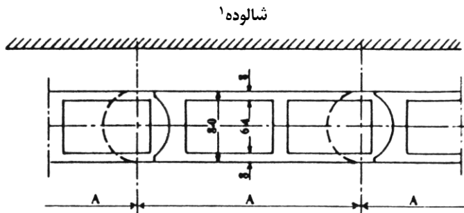
شکل ۵-۶ سپر به طریق دیوار شیاری
