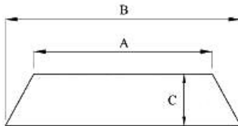
شکل ۱۸-۲- ابعاد ریشه
