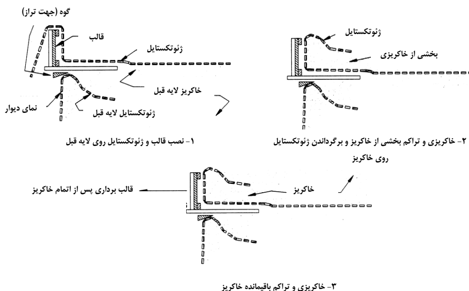
شکل ۲۱-۲۲ مراحل اجرای دیوار خاک مسلح بدون نما
