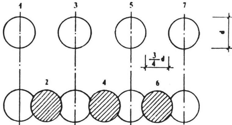
شکل ۶-۳ فاصله بین شمع‌ها، ۷۵/۰ قطر شمع‌ها
