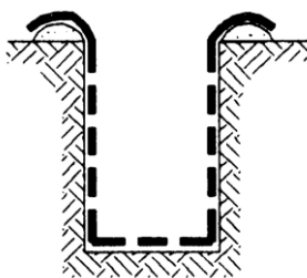
۲- نصب ژئوتکستایل
