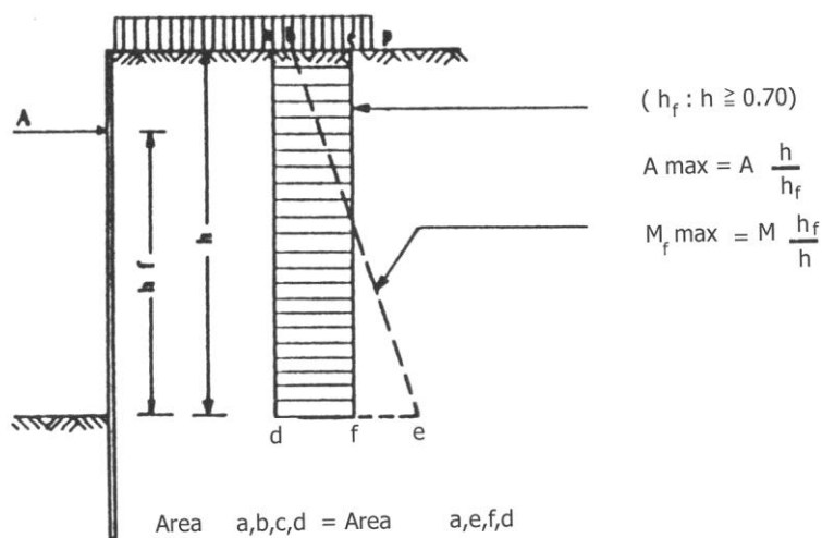
شکل ۶-۷ سپر دارای یک تکیه‌گاه یا یک مهار
