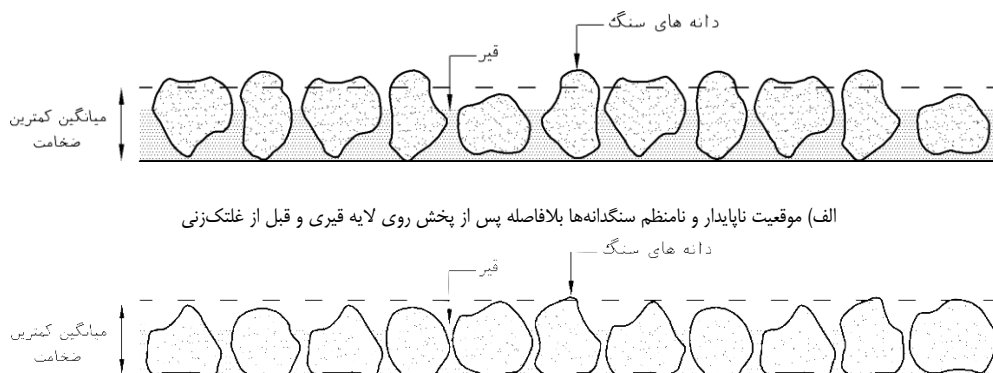
شکل ۱۷-۱ موقعیت سنگدانه‌ها در بستر قیری راه، قبل و پس از غلتک‌زنی و عبور ترافیک
