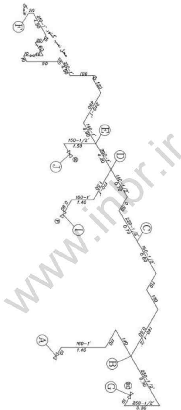
شکل پ-۲-۲ نقشه ایزومتریک لوله کشی گاز نمونه
