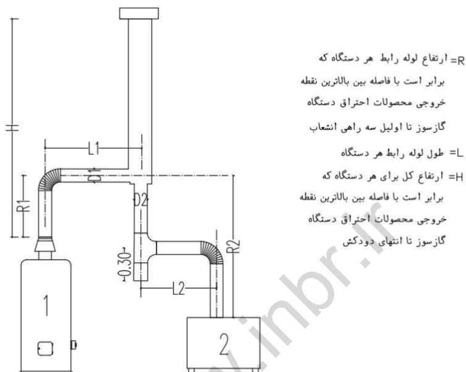
شکل ۴-۱۷-۲ دودکش برای دو یا چند دستگاه گازسوز که در یک طبقه نصب شده‌اند
