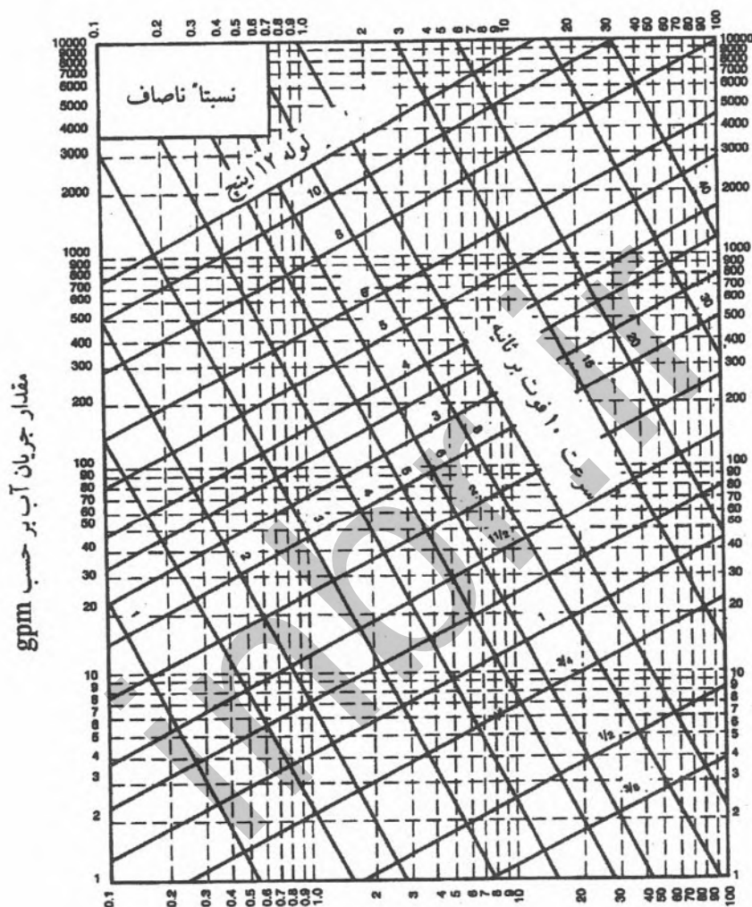
افت فشار آب بر حسب فوت بر اینچ مربع در ۱۰۰ فوت طول
