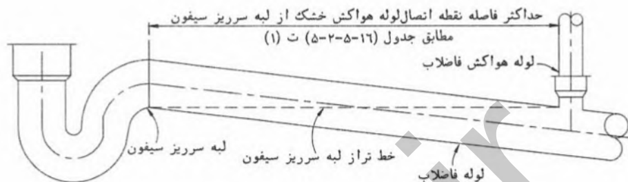
شکل ۵-۲-۱۶ "ت" - اتصال لوله هواکش خشک لوازم بهداشتی
