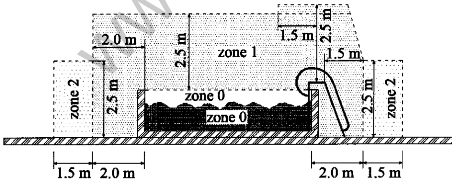
شکل ۱۰-۱۳-۲: طرحواره ابعاد مناطق (zone) برای استخر احداث شده روی کف زمین (دید از کنار)
