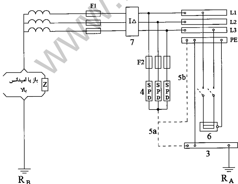
شکل ۴-۱۳-۱-۱۶-۳: طرحواره نصب برقگیر حفاظتی در شبکه توزیع سیستم نیروی IT
