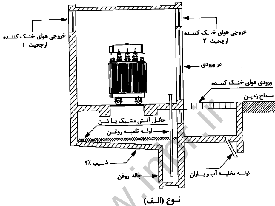
شکل ۵-۱۳-۳-۲:۳ (نوع الف) - طرحواره مقطع قائم اتاق ترانسفورماتور روغنی با تهویه مکانیکی و هم سطح زمین
