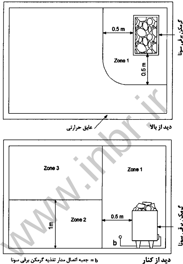
شکل ۱۳-۱۰-۶ طرحواره مناطق (zone) مربوط به سونا بر اساس درجه حرارت محیط آن
