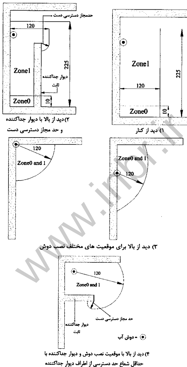
شکل ۱۳-۱۰-۴-۲: طرحواره موقعیت و ابعاد مناطق (zone) ها در حمام بدون زیردوشی
