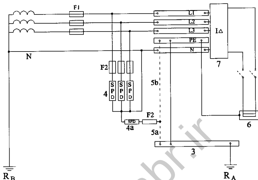
شکل ۳-۱۳-۱-۱۶-۳: طرحواره نصب برقگیر حفاظتی در شبکه توزیع سیستم نیروی TT با قرارگیری برقگیر حفاظتی قبل از کلید حفاظتی جریان باقی‌مانده (RCD)
