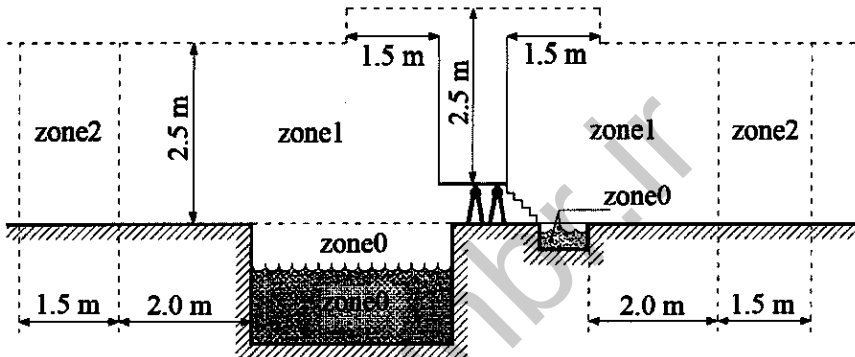
شکل ۱۰-۱۳-۵: طرحواره ابعاد مناطق (zone) برای استخر و تخت پرش (دید از کنار)
