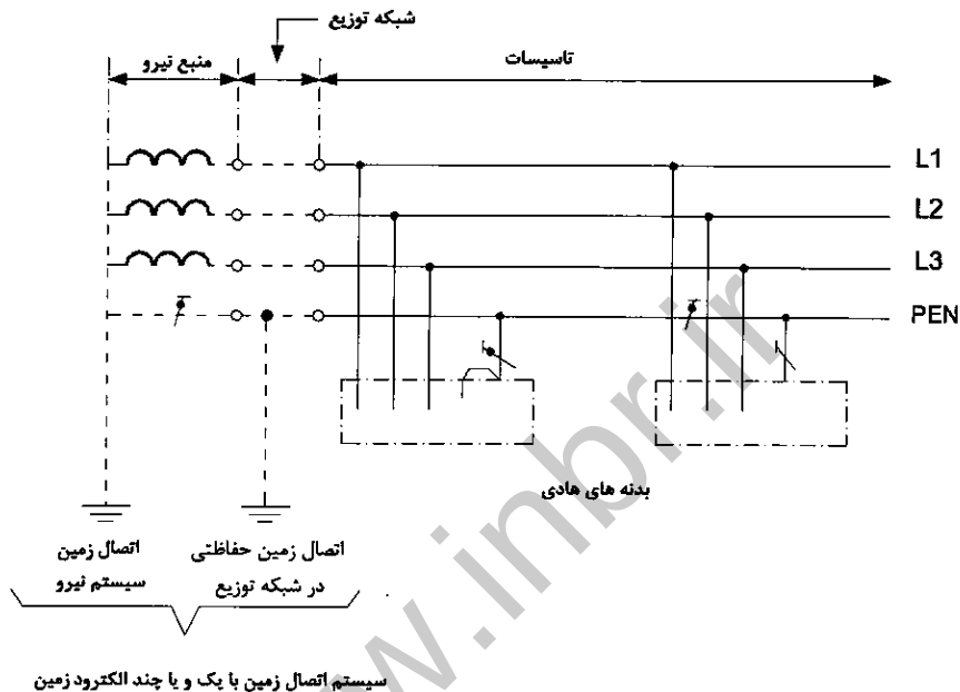
شکل پ ۱-۱-۲ سیستم TN-C در سیستم سه فاز چهار سیمه با هادی مشترک حفاظتی - خنثی در سرتاسر سیستم
