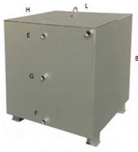
شکل ۴- مخزن انبساط باز ابعاد مخزن چهار گوش طبق جدول روبه رو ساخته می شوند.
