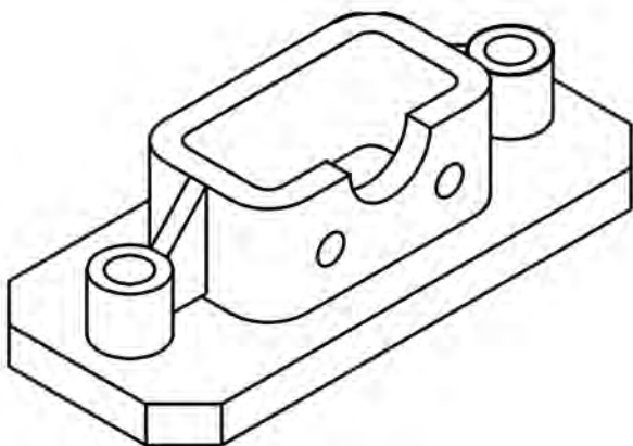
شکل ۳-۳۵- پایه
