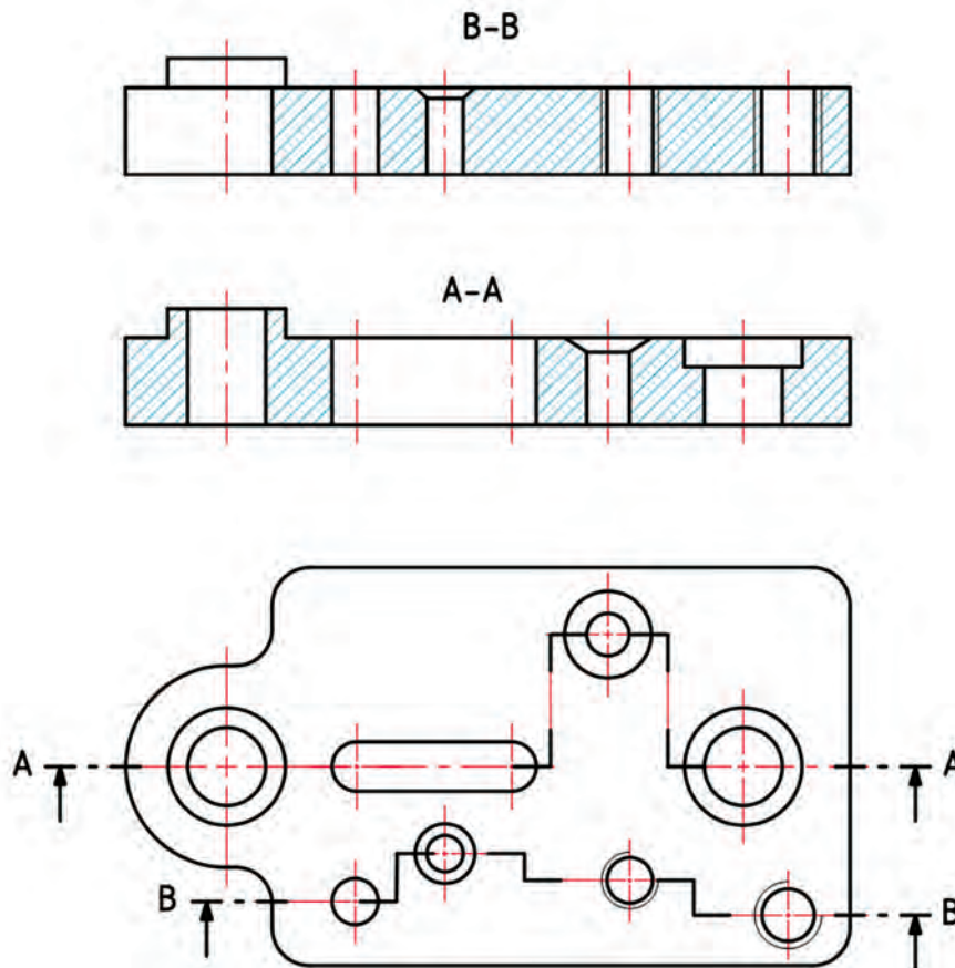
شکل ۳-۴۲- پایه چدنی
