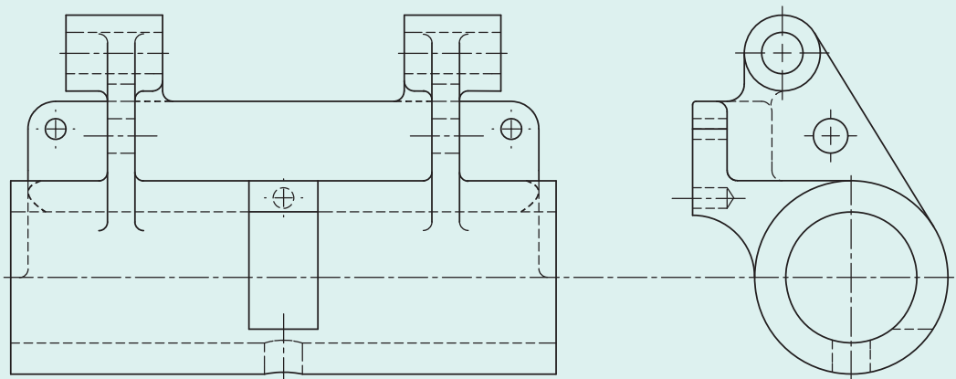
شکل ۴-۴۶، دیوارکوب
