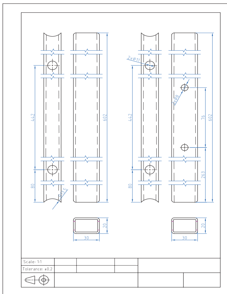
شکل ۵۵-۲ نقشه سوراخ کاری قطعات پایه
