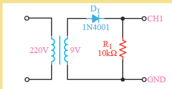
شکل ۱-۱۷ آداپتور
