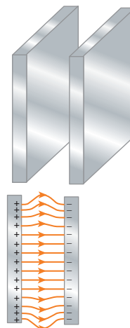
شکل ۲۰-۱ طرحی از خطوط میدان یکنواخت بین دو صفحه رسانای موازی با بارهای هم‌اندازه و ناهمنام
