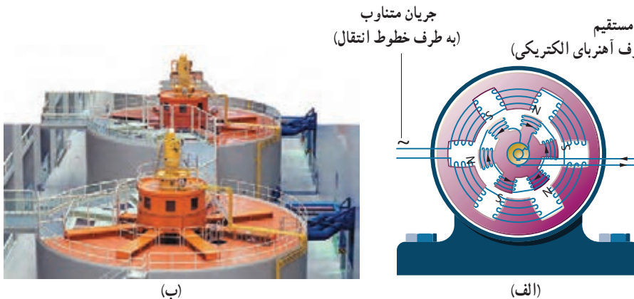
شکل ۳-۳۶ الف) در مولدهای صنعتی با چرخیدن آهنربای الکتریکی بین پیچه‌ها، جریان متناوب تولید می‌شود. ب) نمایی از مولدهای صنعتی تولید برق.
