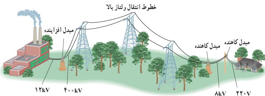
شکل ۳-۳۷ قبل از انتقال توان الکتریکی از نیروگاه‌ها، مبدل‌های افزایشنده، ولتاژ را تا حدود 400 \text{ kV} افزایش می‌دهند. در انتهای مسیر، مبدل‌های کاهشنده، ولتاژ را کاهش می‌دهند تا توان الکتریکی با امنیت بیشتر به محل مصرف برسد.
