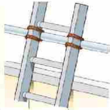
اشکال ۷- نحوه تکیه‌گاه نردبان از یک طرفه
