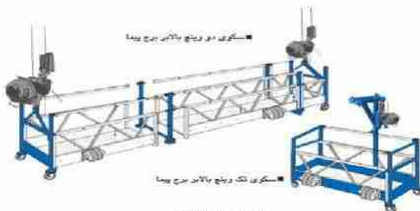
انتهال ۱۲۱- جایگاه کار آویزان
