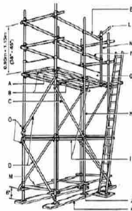
شکل ۴۶ - داربست با کلمه اجزاء
