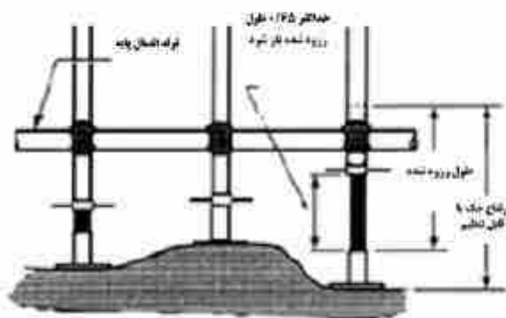
انکال ۵ - نحوه برپایی داربست
