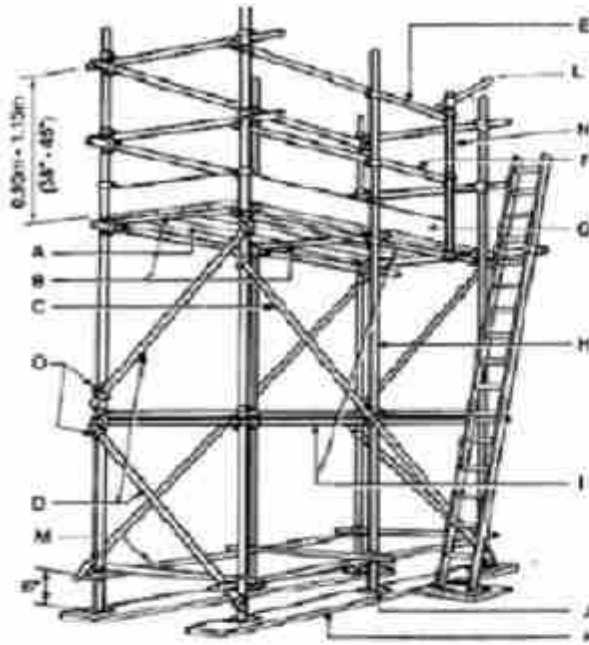
شکل ۴۶ - داربست یا کلبه اجراء
