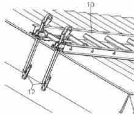
شکل ۳- تودبان دو طرفه
