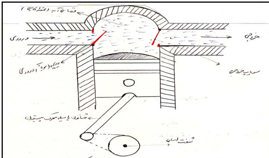
شکل (a-2) شکل ساده پمپ پیستونی نوع فشاری یکطرفه (یک عمله) در حالت عادی
