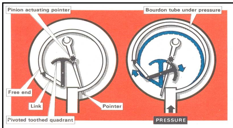
طرح های ساده شده مکانیزم فشار لوله بوردون یا شاخص خلاء
