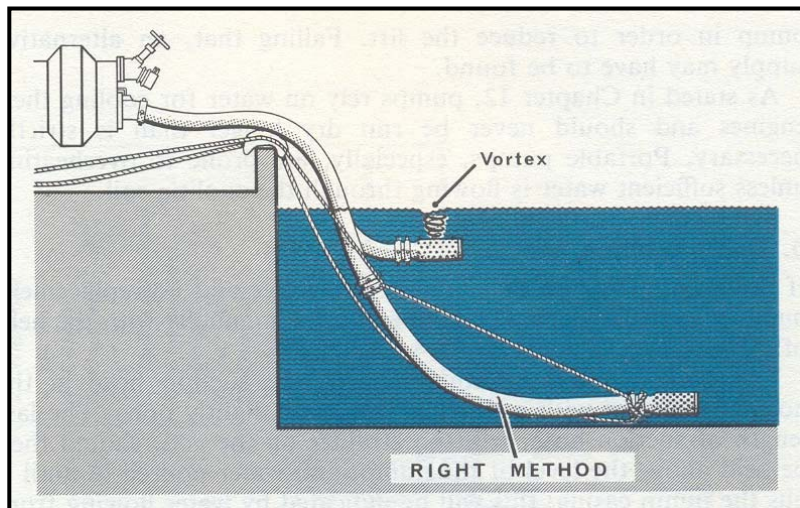
طرح نمایش تشکیل شدن کیسه های هوایی به علت قرار گرفتن صافی خرطومی در نزدیکی سطح آب
