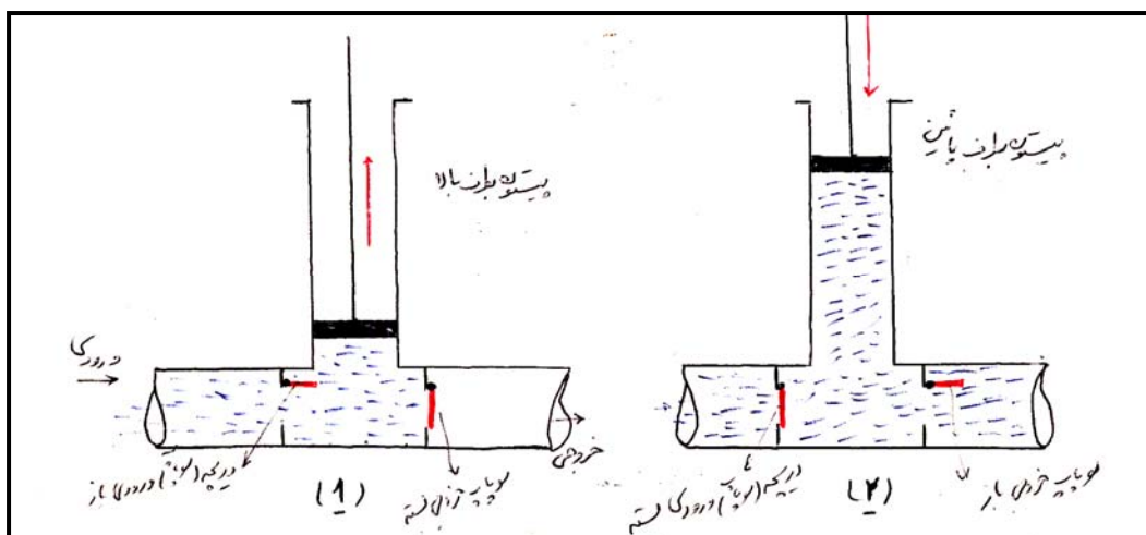
شکل (b-2) پمپ پیستونی فشاری یکطرفه (یک عمله) در دو حالت عملکرد
