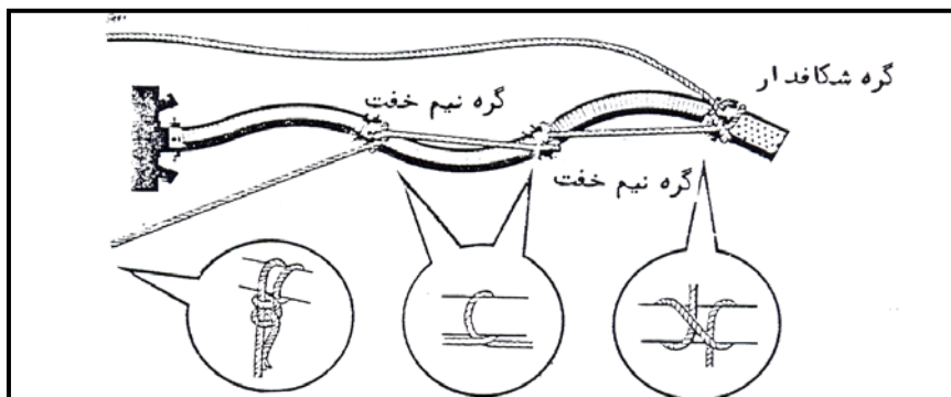
طناب را به وسیله بستن یک حلقه و دو گره نیم خفت به یک شی ثابت محکم ببندید.
