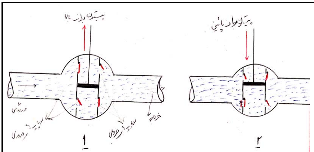
شکل (c - 3) سیکل عملکرد دو حرکت یک پمپ فشاری دو عمله پیستونی را نشان می دهد.
