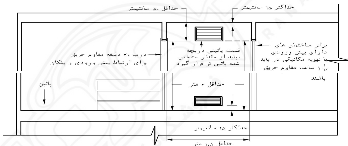
جزئیات اجرای کانال ها و دریچه های سامانه تهویه لابی
